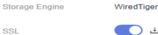
Figura 9-2 Ativar SSL
