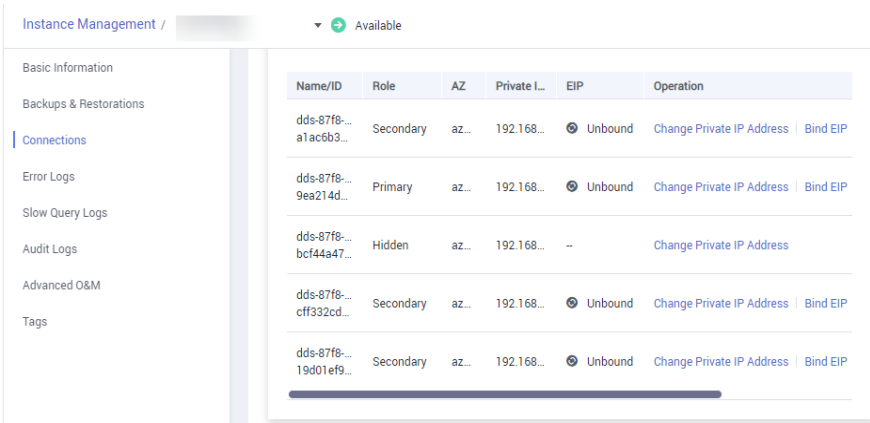
Figura 11-2 Conexões
