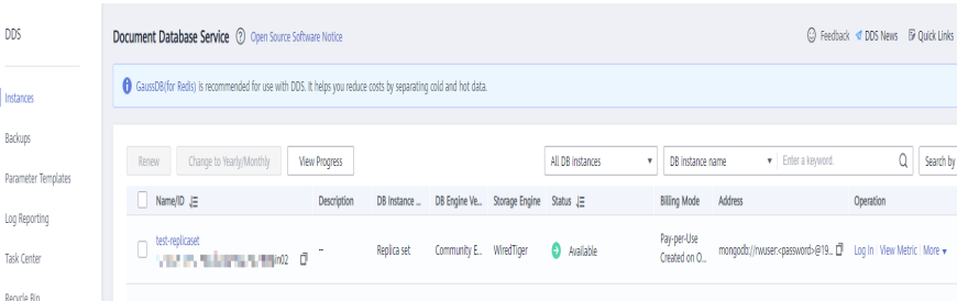
Figura 11-1 Instâncias
